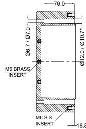
SECTION A-A
